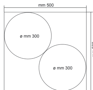
Piano di cottura in pietra refrattaria Refractory brick deck.
