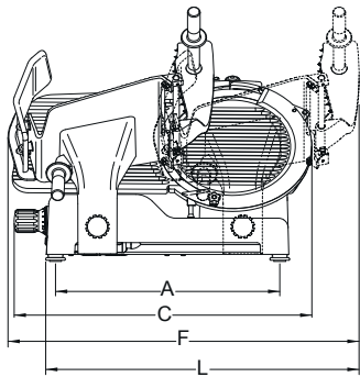
Gambe opzionali Optional legs
